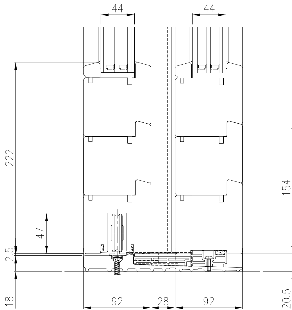
SEZIONE VERTICALE
